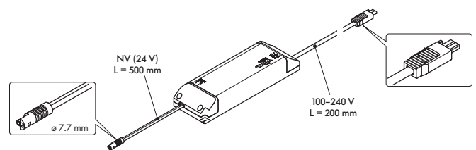
Fig. 2: Converter
